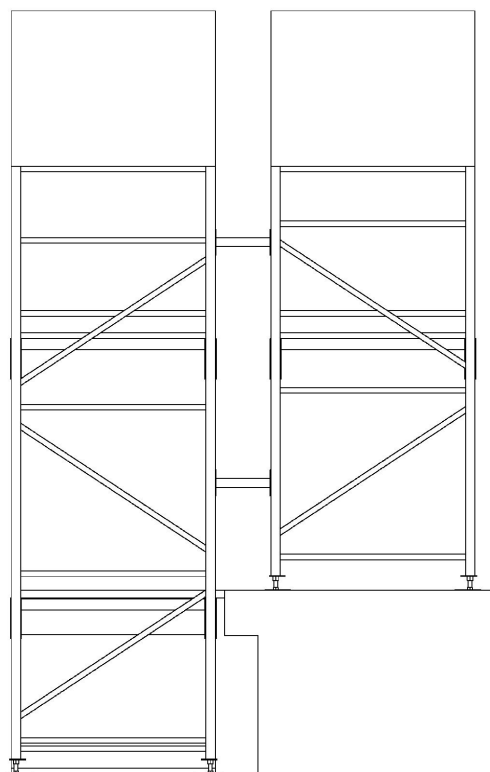
【使用状態を示す参考右側面図】
