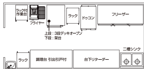
厨房スペース基本レイアウト
