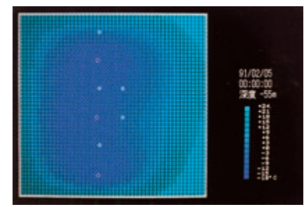
凍土の温度シミュレーション
