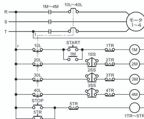
図3 順序始動・順序停止制御の回路例
