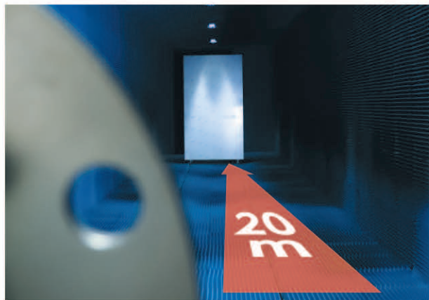
写真「Waveラボ」内の電波暗室
