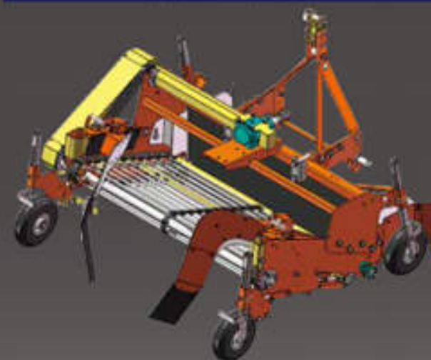
角棒タイプ(新型)
