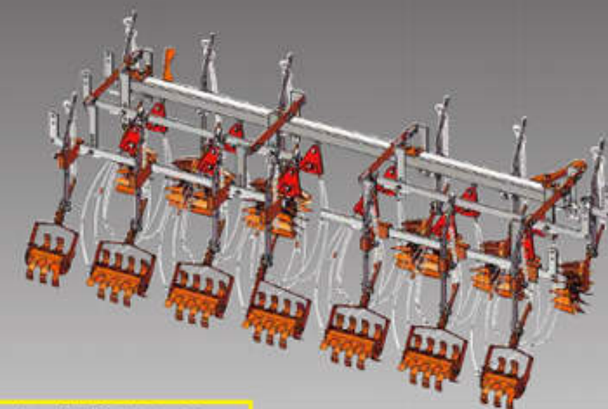
米輪・レーキ・ガス抜きローター
