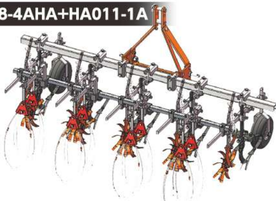
深耕カッター・ゴロださん・レーキ+玉輪L5条(玉ねぎ用)
