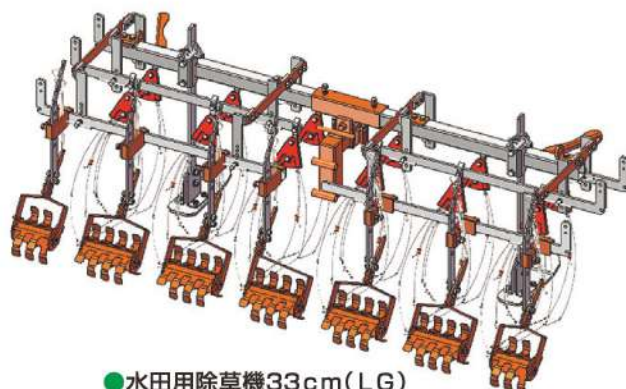
●水田用除草機33cm(LG) ガス抜きローターB・レーキ
