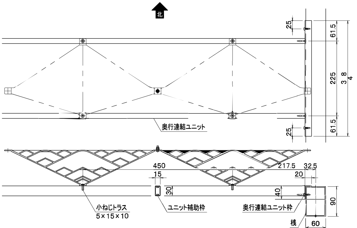
奥行連結ユニット 平面・正面図
