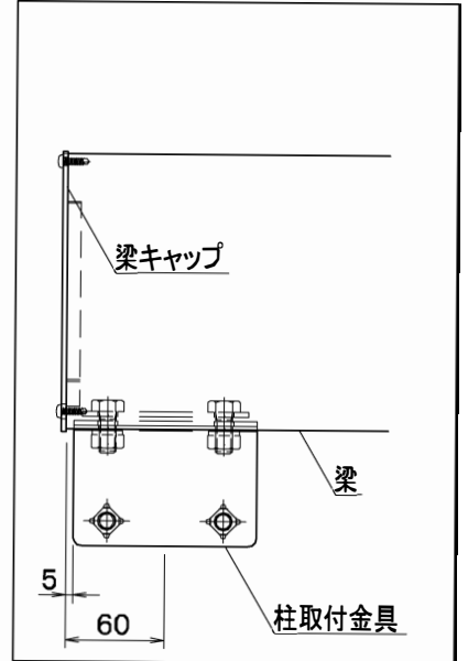
■納まり図
