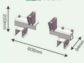
受注生産 みのる用ヒッチ (RX4用) 水田
