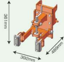
イセキ用ヒッチ (アイサイカ用)
