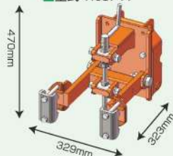
三菱用ヒッチ (MPR65用)
