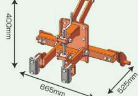
ヤンマー用ヒッチ (RG用)
