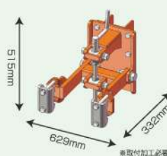
田植機用ヒッチ
