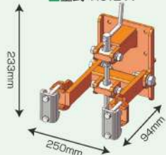
受注生産 みのる用ヒッチ (LTR・LRM用) 水田
