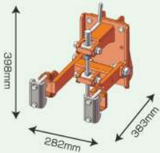
ヤンマー用ヒッチ (MD14用) (MD20用)
