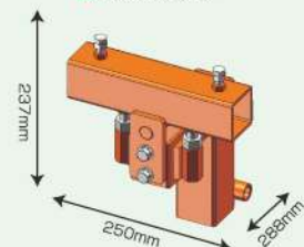
受注生産 みのる用ヒッチ (LTR・LRM用) 水田
