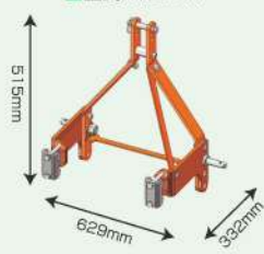
三点ヒッチM ■型式:H601-A
