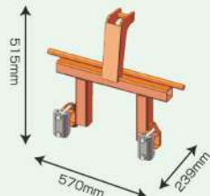
ヤンマー用ヒッチ (アグリカ用)
