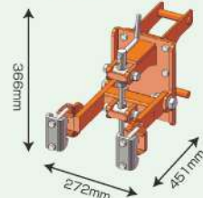
受注生産 みのる用ヒッチ (RT31・32)
