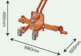
クボタ用ヒッチ (NS67用)
