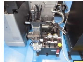
圧油・潤滑兼用 ポンプユニット (オーバーホール)
