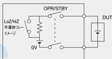
LoZ/HiZ: サスペンド時の出力抵抗切替 OPR/STBY: オペレート/スタンバイ切替リレー 出力状態の概念図
