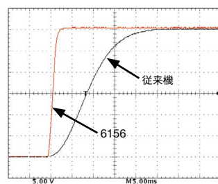
出力レスポンス波形 (0V→30V)
