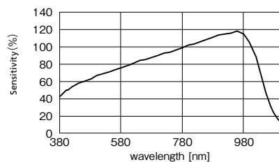
82311B/82321B 波長感度特性
