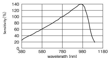
82313B/82323B 波長感度特性
