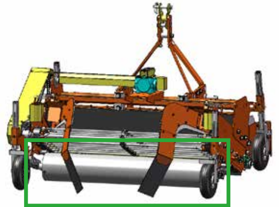
本体部取付位置 (左)
