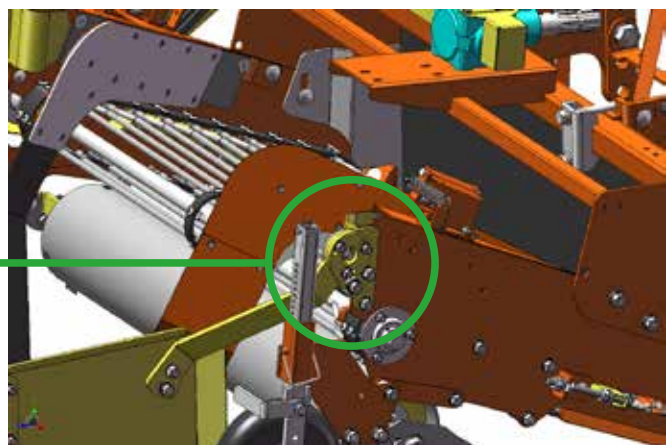
本体部取付位置 (右)
