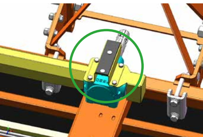
収納台 ASSY 取付
