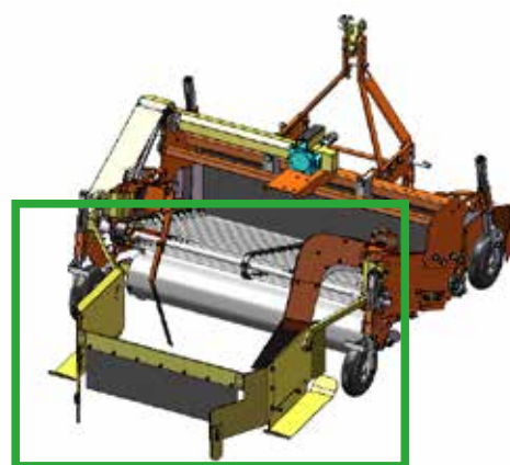
本体部取付位置 (左)
