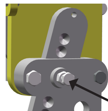
ネジで高さを調整
