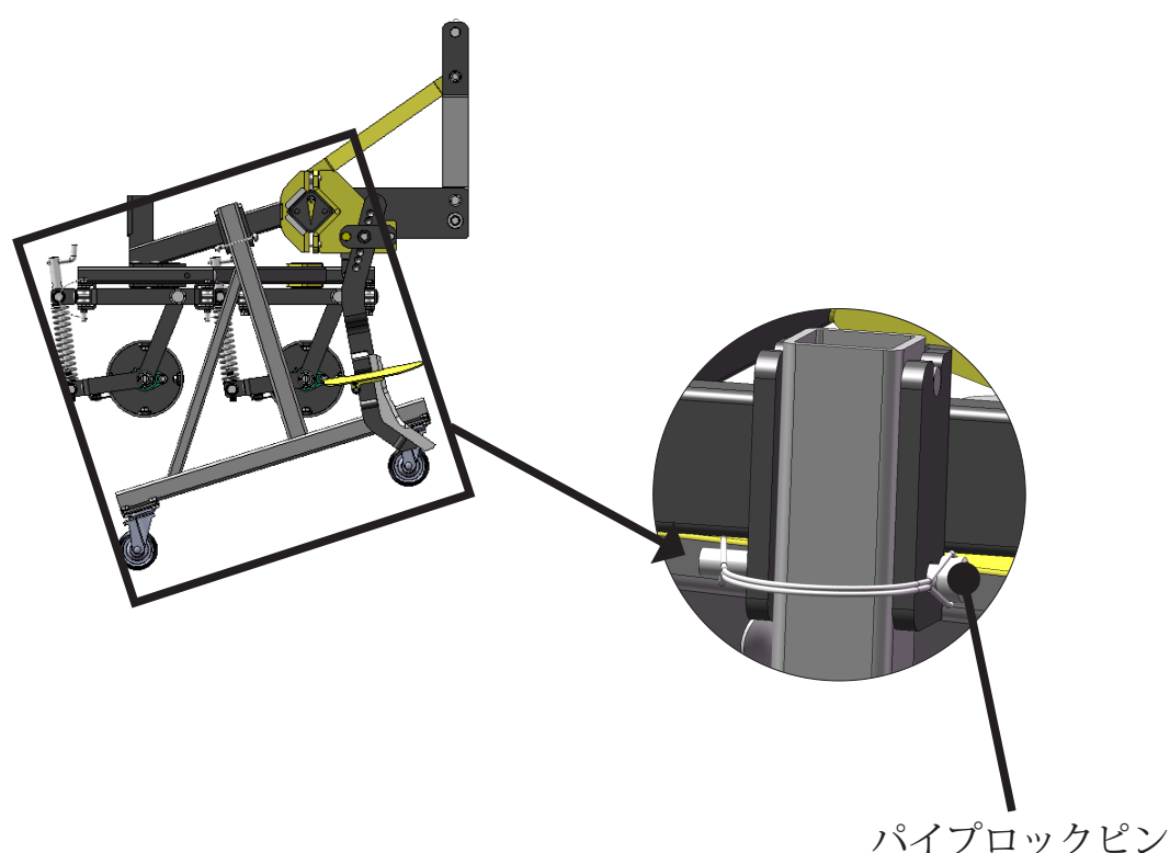
前方スタンド
