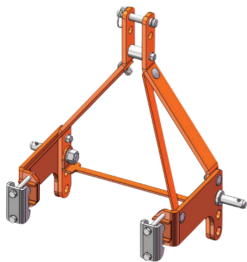
3点ヒッチ M
