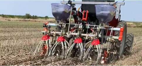
施肥機（アグリテクノ矢崎）ホース 2 本タイプ（接地輪）
