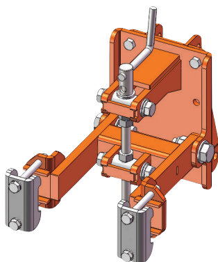
クボタ用ヒッチ (SPU 用)
