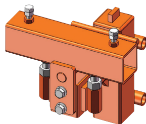
みのる用ヒッチ (RX4 用) 水田
