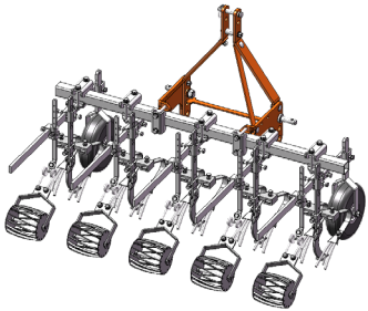
今回使用した新玉除草カルチ 型式：H018-4BHA
