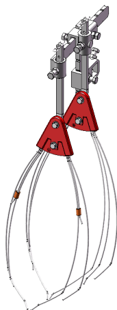
商品名：後付レーキセット 型式：H018-4H ※ 4 畦分
