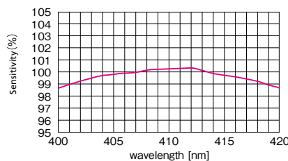
82314B/82314BW/32324B 波長感度特性 (405nm)
