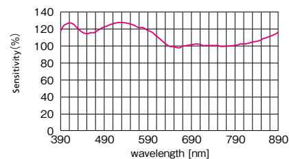
82314B/82314BW/32324B 波長感度特性 (全帯域)
