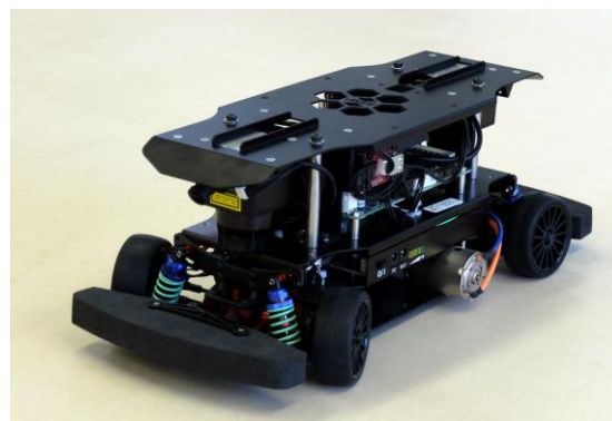
実車 1/10 スケールロボットカー RoboCar 1/10
